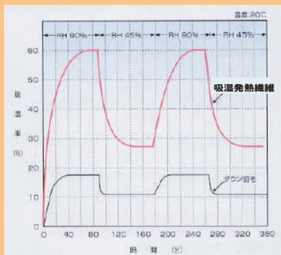
特殊吸湿発熱繊維の吸放湿曲線
